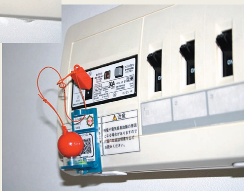
▲感震ブレーカー（簡易型）の写真▶
